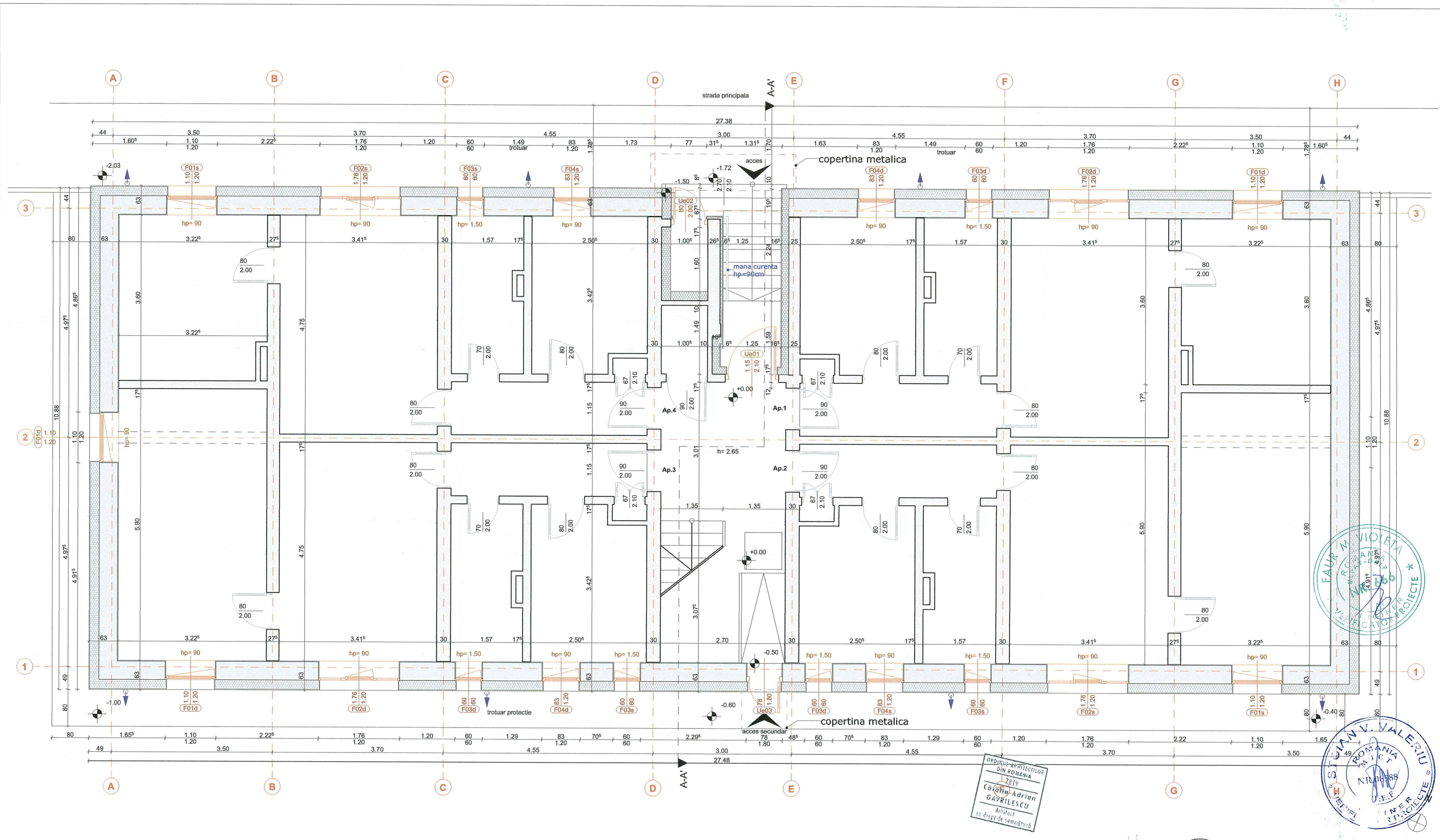
Plan parter - propunere SC 1:50
