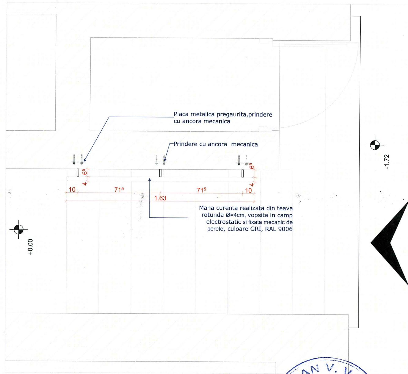
Plan CM_M1 SC 1:20
