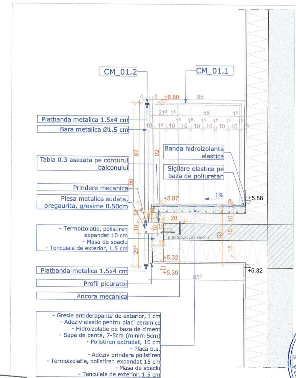
Secțiune CM_01 SC 1:20
