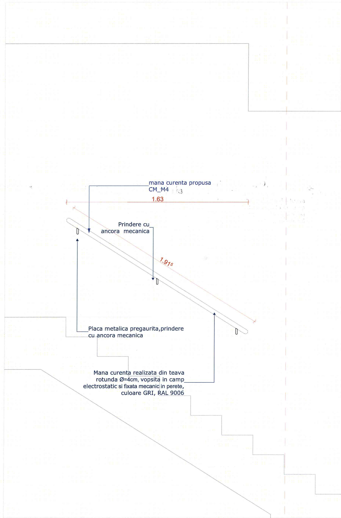
Vedere CM_M1 SC 1:20
